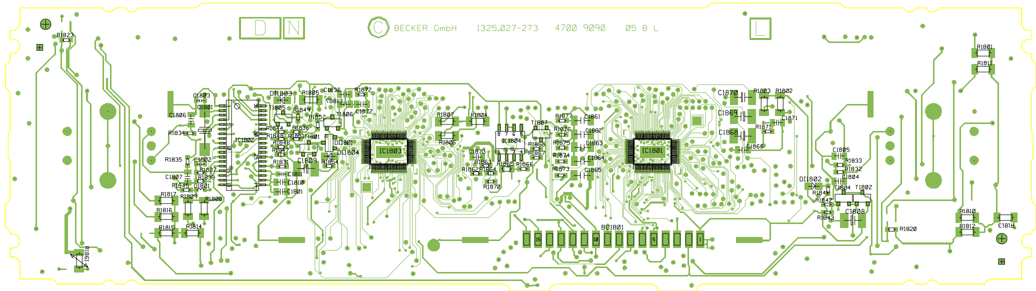
Lötseite
