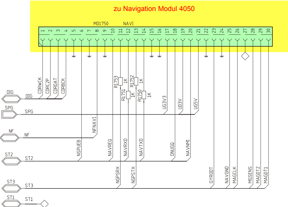
Pinbelegung NaviBoard Pin 1 Richtung Konnektor
